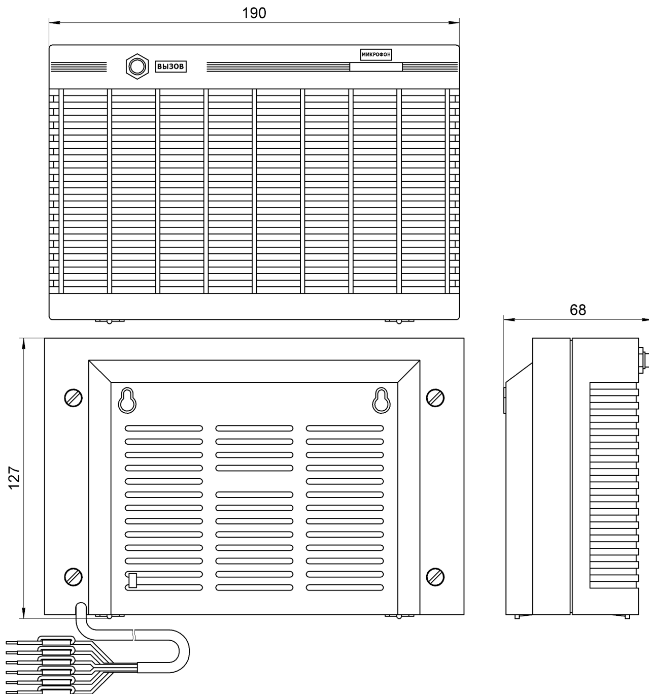
Рис.1 Внешний вид Устройство громкоговорящей связи УГС-014 НШЕК.465112.014
